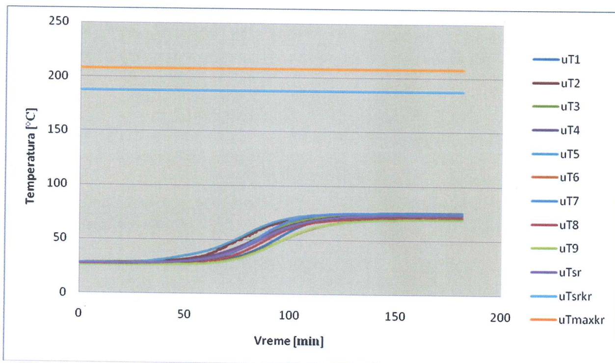
Slika 3 - Vremenske promene temperatura na neizloženoj površini uzorka (termoparovi za srednju vrednost temperatura)
