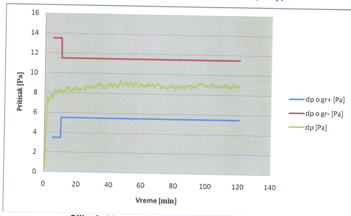
Slika 2 - Vremenska promena pritiska u ispitnoj peći
